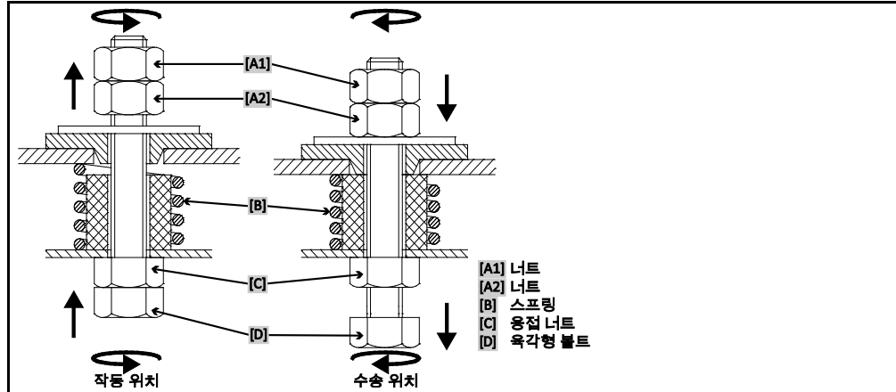
수송 잠금 장치의 그림
