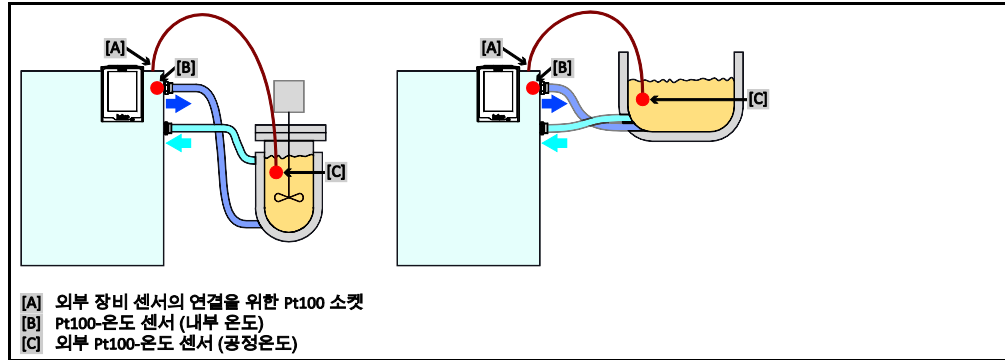
스키마 온도 제어 시스템
